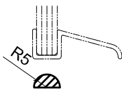
Acryl-Dichtprofil zur zusätzlichen Abdichtung bei ungünstigen Wannensituationen Art.-Nr.: 04.5500
